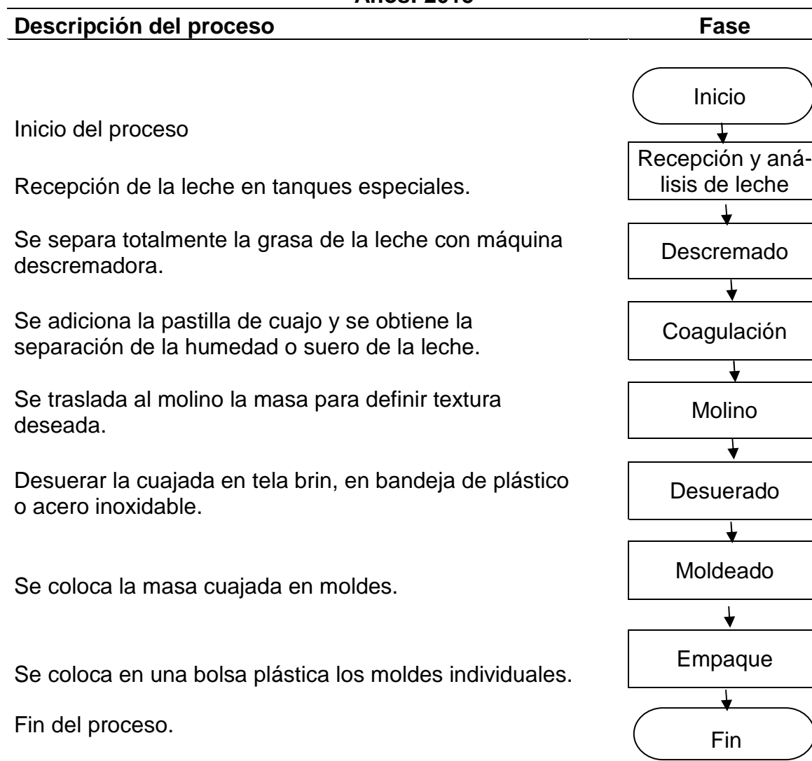
Grafica 4 Municipio de La Libertad, Departamento de Petén Producción de Lácteos Flujograma del Proceso Productivo de Queso de Capa Años: 2015
