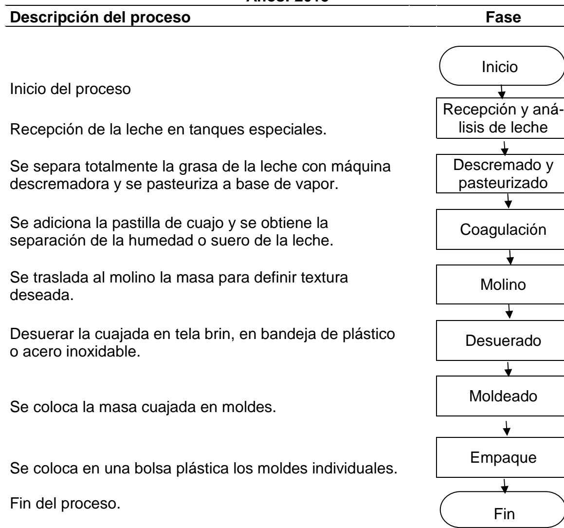
Grafica 3 Municipio de La Libertad, Departamento de Petén Producción de Lácteos Flujograma del Proceso Productivo de Queso Pasteurizado Años: 2015
